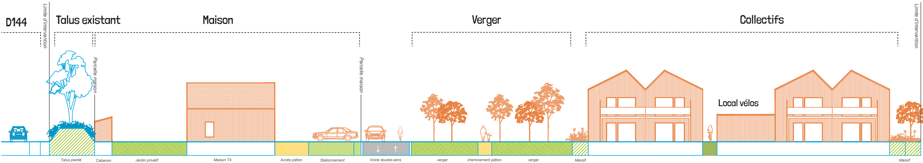
Coupe Est-Ouest
